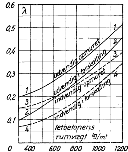
Fig. 3. Varmeledningstal for letbeton i blokke eller plader.
